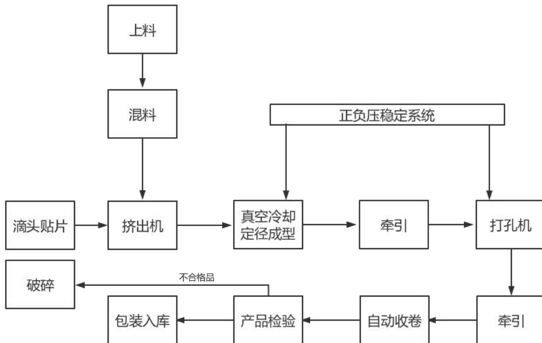
图 2 滴灌管（带）生产工艺流程图
